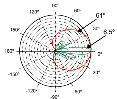
UMTS pattern per sector
